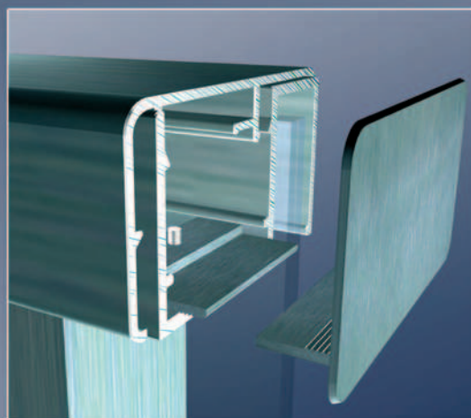
DETALLE TAPA SUPERIOR
